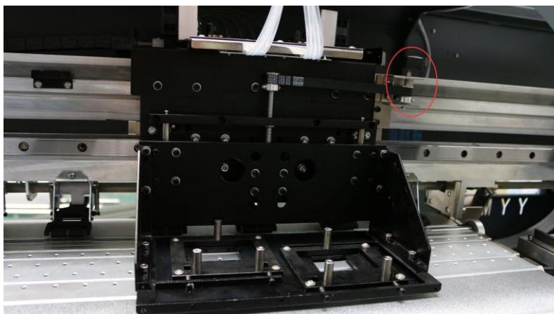
PC3200 调整喷头高低
