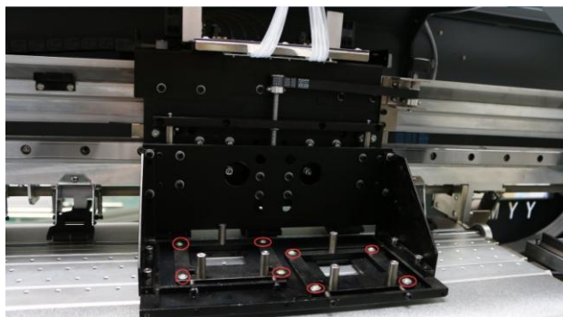
PC3200 喷头的调整位置（红圈）
