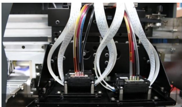
PC3200 喷头墨囊（墨囊集成在喷头内部）
