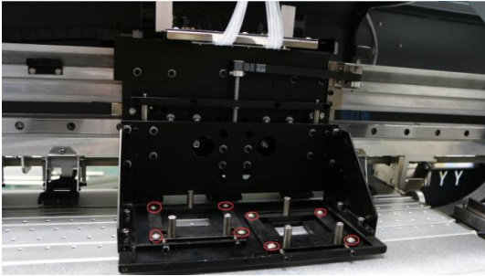
PC3200 喷头的调整位置（红圈）
